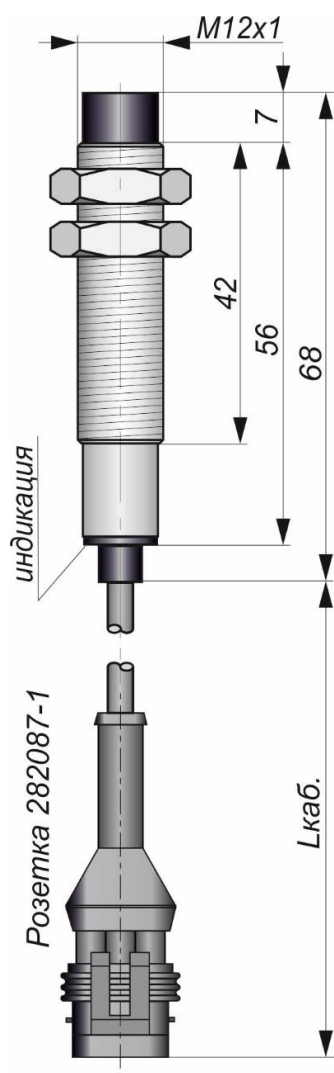
Габаритный чертеж
